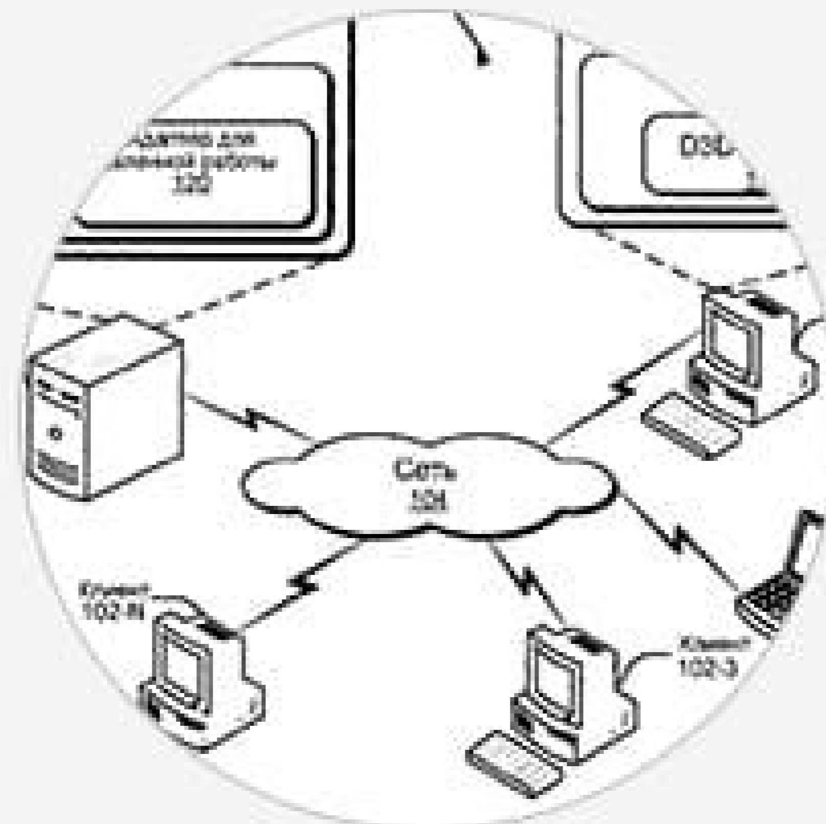
Архитектура программы
